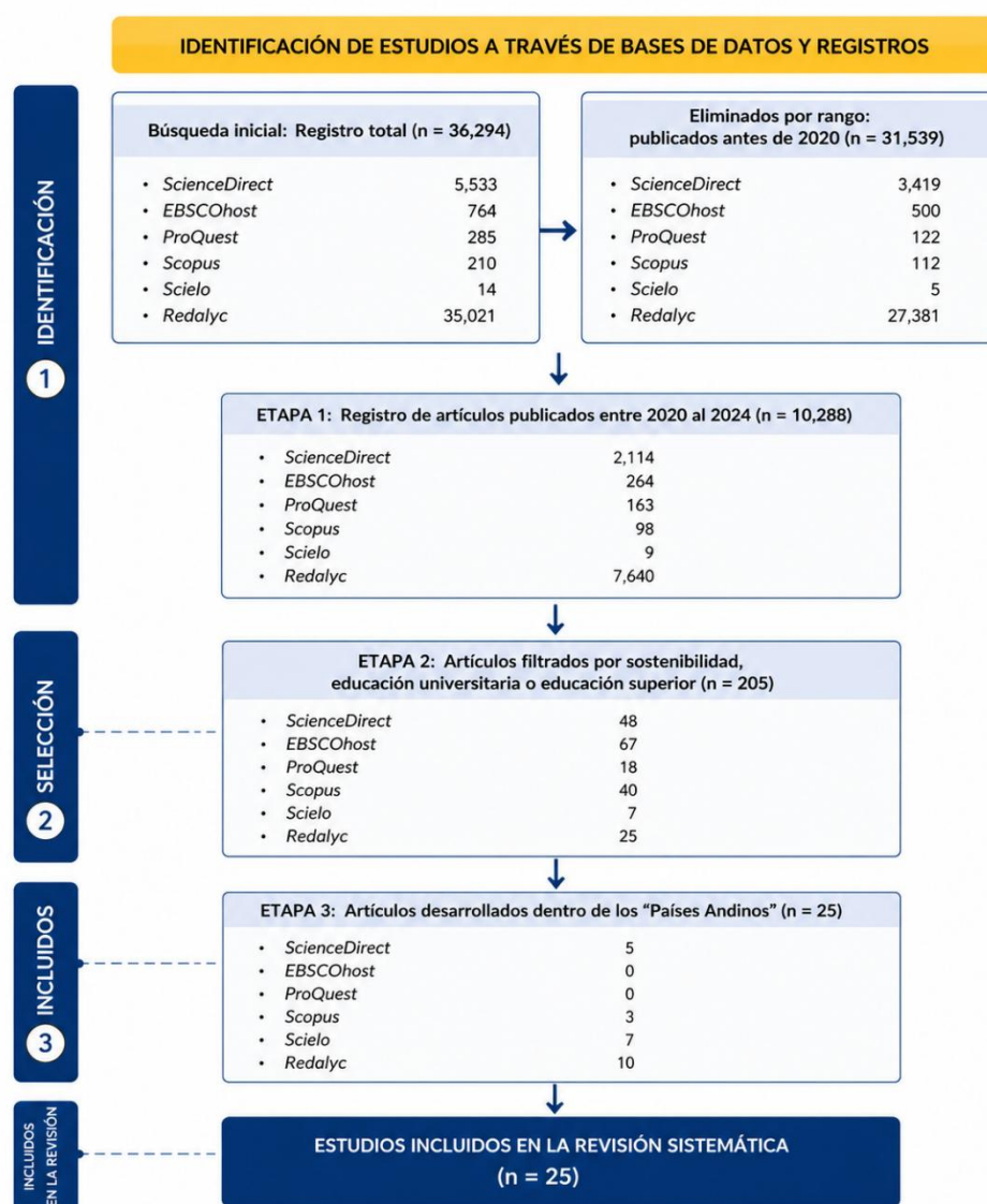
Figura 1. Diagrama de flujo según la norma Prisma
